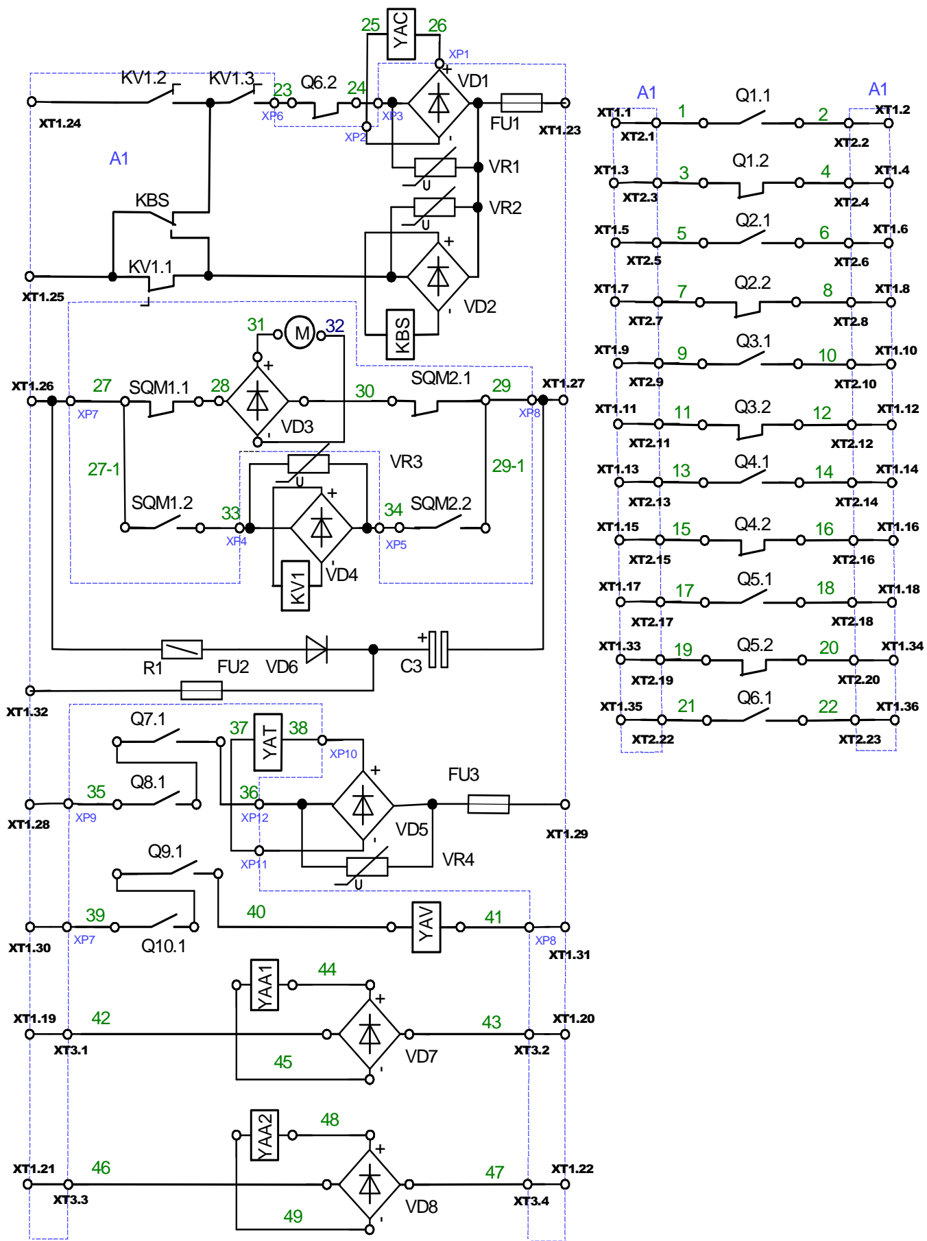
Схема электрическая принципиальная Рис.4
